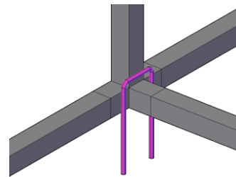
Tilladt fastgørelse af hoop uden afstandstykke
