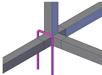
Tilladt fastgørelse af hoop uden afstandstykke
