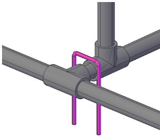
Tilladt fastgørelse af stakit m/afstandstykke
