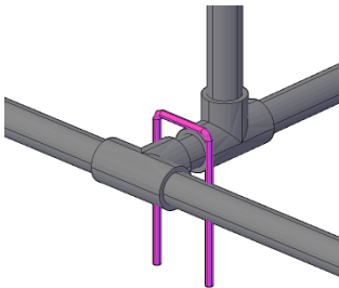
Tilladt fastgørelse af hoop m/afstandstykke
